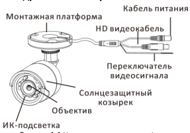
Рисунок 1-1 Цилиндрическая камера I типа
