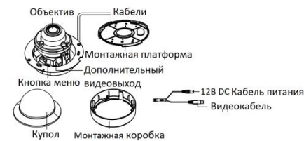
Рисунок 1-14 Купольная камера III типа
