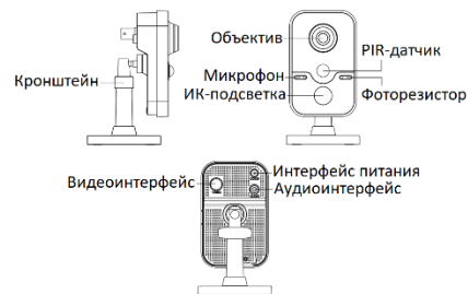
Рисунок 1-26 Компактная камера
